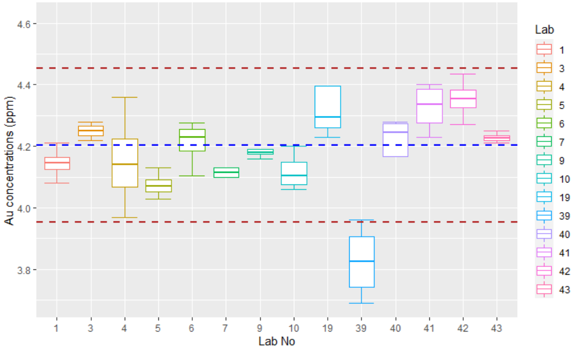
PBS-88 Au Box Plot
