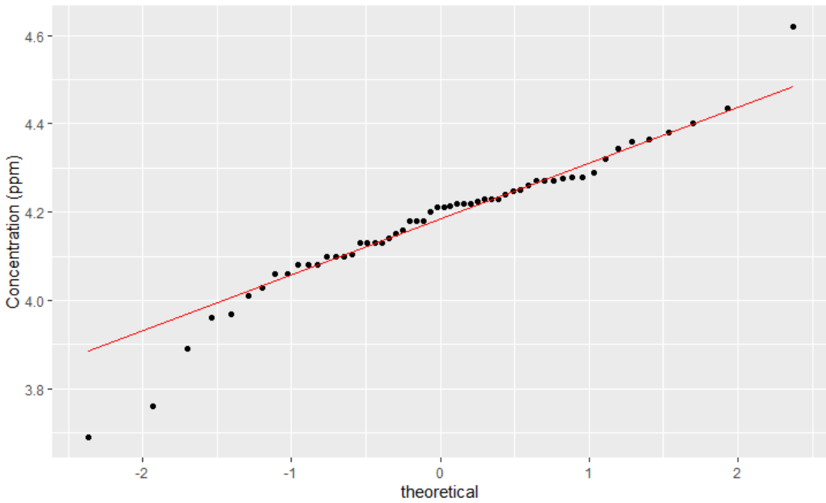
PBS-88 Au Q-Q Plot
